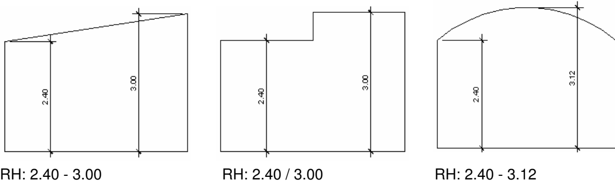
Abbildung 5: Beispiel Räume mit verschiedenen Höhen
