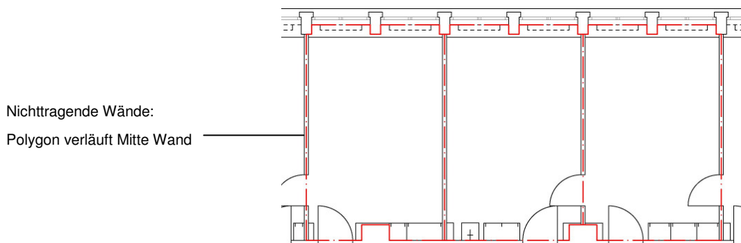
Abbildung 16: Polygonverlauf bei nichttragenden Wänden (Wände d < 15 cm)
