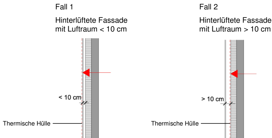
Abbildung 17: Messebene der thermischen Hülle bei hinterlüfteten Fassaden
