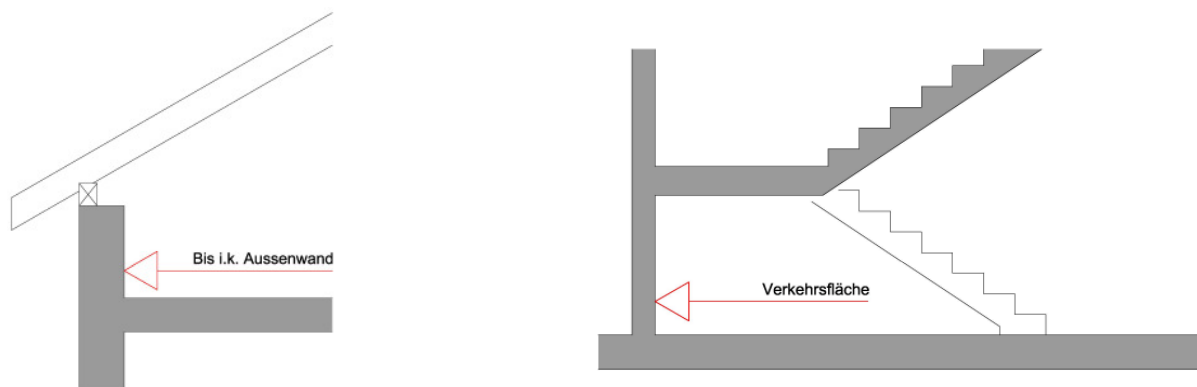
Abbildung 4: Behandlung von Räumen unter Steildächern und unter Treppenläufen
