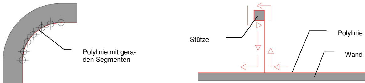
Abbildung 11: Polygone ohne Bögen und Einbinden von Stützen in Polygone
